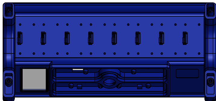
HyPro-Oberteile 8MSA1/Farbe: blau TNr.: 3.300.1125
