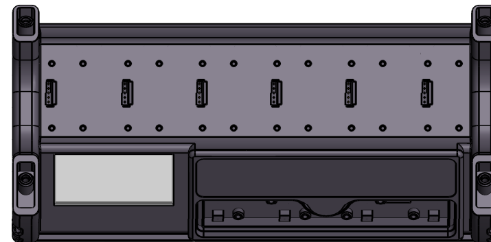
HyPro+-Oberteil 6MSA1 / 2TB TNr.: 3.300.1181
